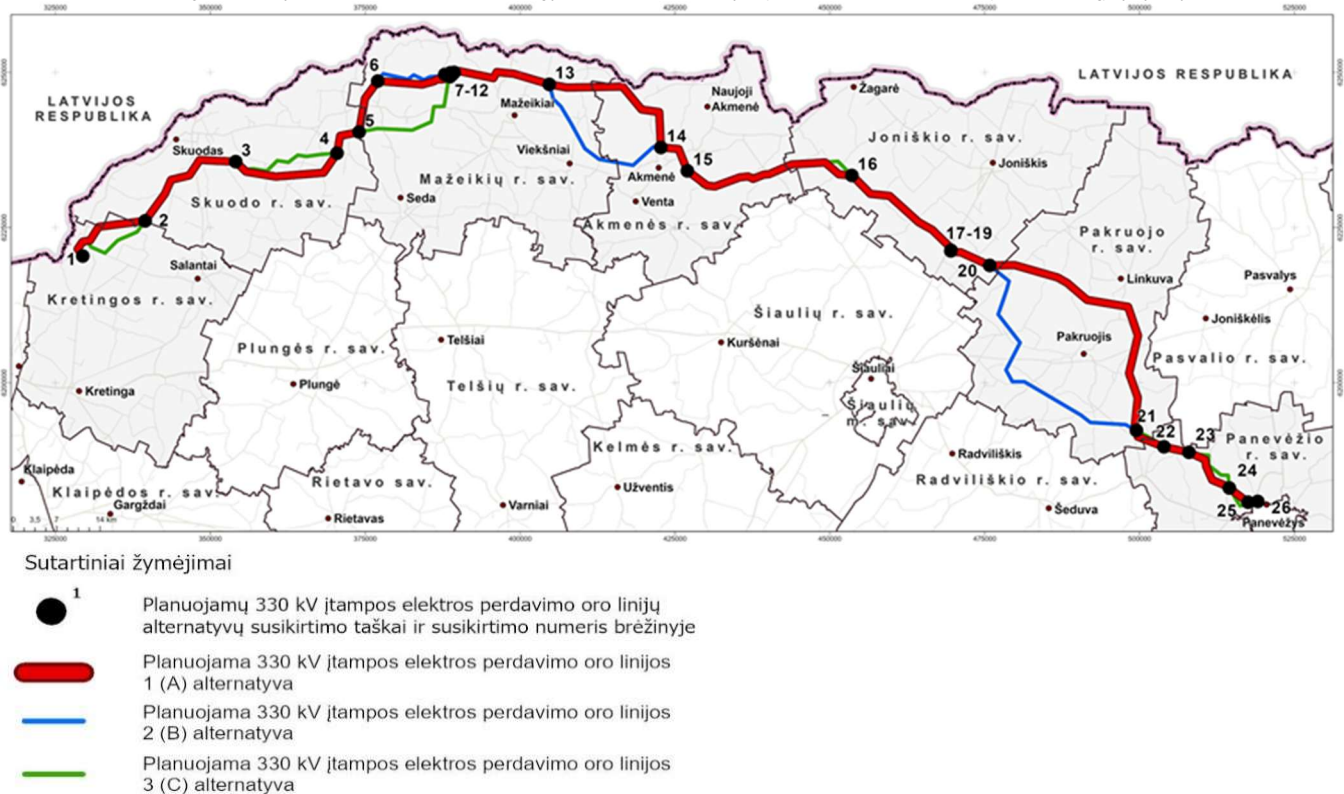
4 pav. Preliminarios 330 kV elektros perdavimo oro linijos trastos alternatyvos (A) schema
