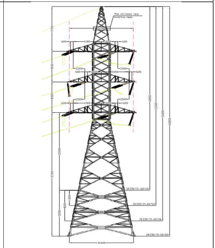
4.7.4 pav. 330kV dviejų grandžių inkarinė atrama
