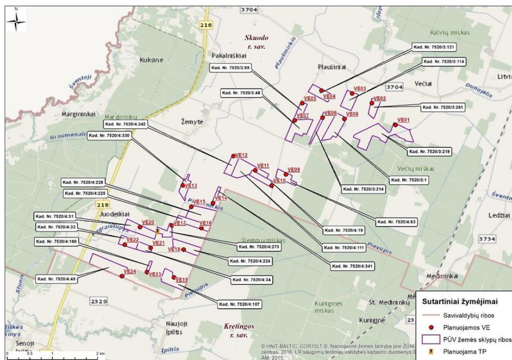
3.1.1 pav. PUV vietos situacinė schema.
