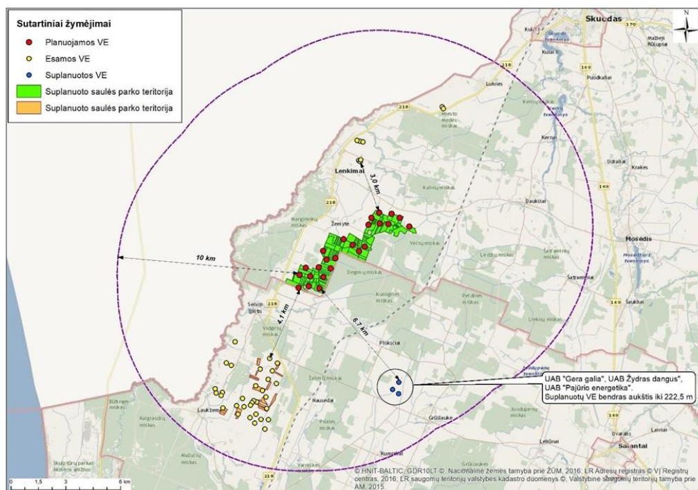
3.2.3 pav. PUV teritorija gretimų VE parkų atžvilgiu.
