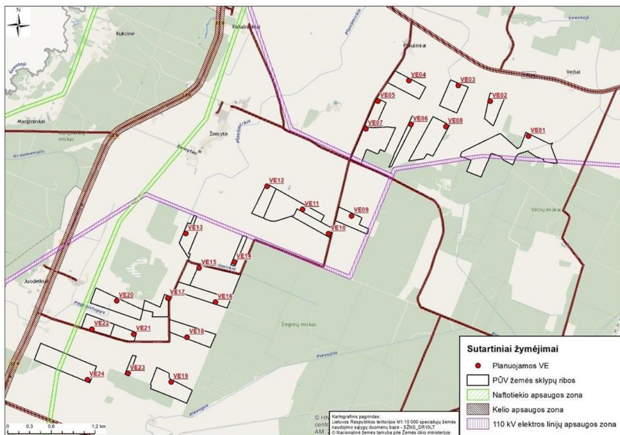
3.2.3 pav. Planuojamų įrengti VE, gretimų bei išterpiančių žemės sklypų išsidėstymas.
