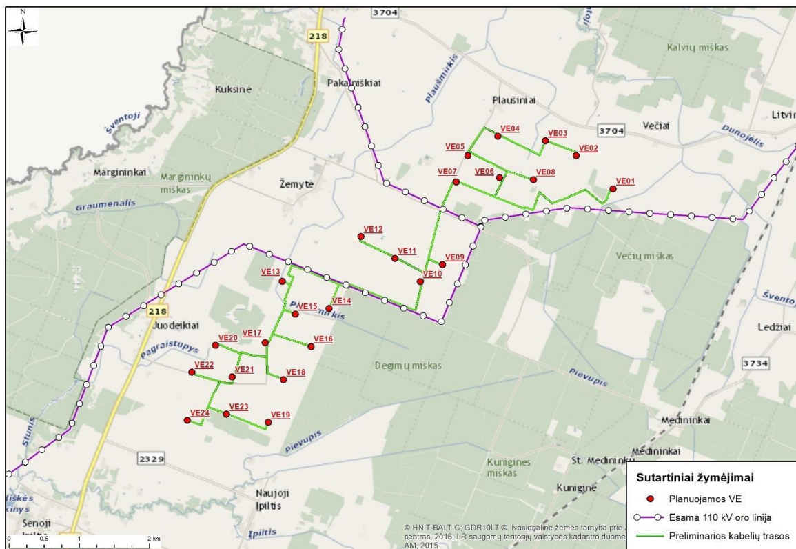
2.2.1 pav. Esama ir planuojama inžinerinė infrastruktūra, preliminaros planuojamų požeminio kabelių trasos.
